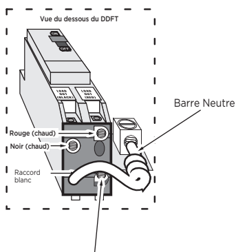
Câble blanc vers le spa
