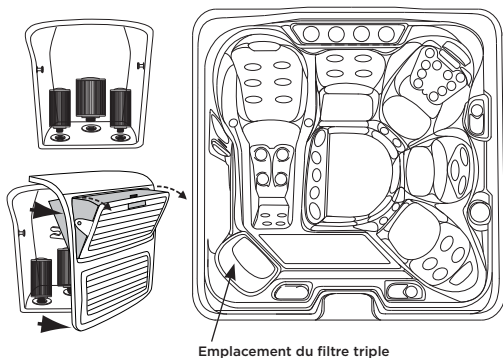
Emplacement du filtre triple
