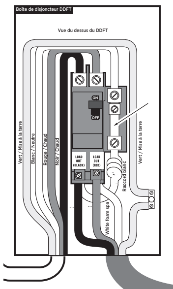
Câble blanc vers le spa
