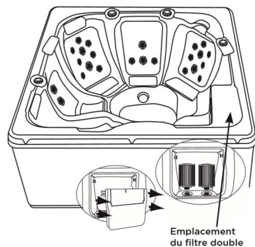
Emplacement du filtre double
